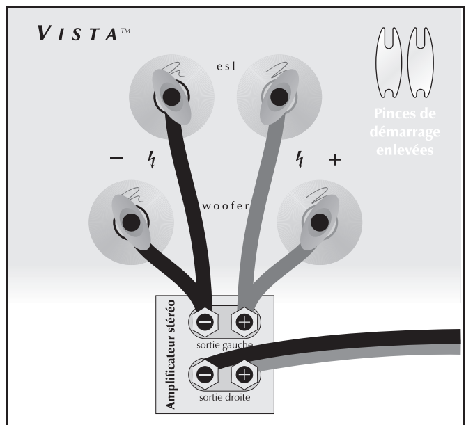
Figure 3. Raccord à deux fils. Un canal illustré.
