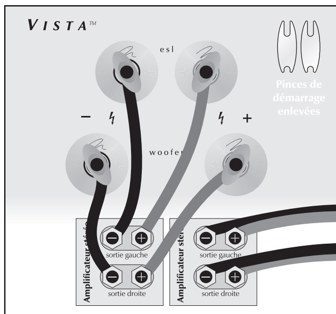
Figure 5. Raccordement par bi-amplification verticale. Un canal illustré.
