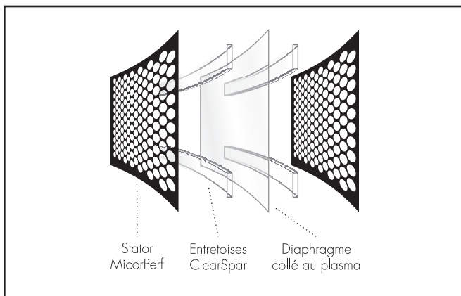
Figure 15. Vue en coupe d'un transducteur électrostatique XStat™. Remarquez la simplicité due au petit nombre de pièces utilisées.
