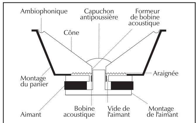
Figure 16. Vue en coupe d'un haut-parleur à bobine en mouvement typique. Remarquez la complexité due au grand nombre de pièces utilisées.
