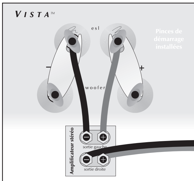
Figure 2. Raccord à un fil. Un canal illustré.
