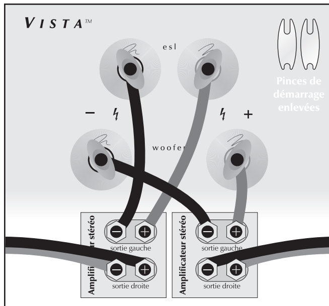
Figure 4. Raccordement par bi-amplification horizontale. Un canal illustré.
